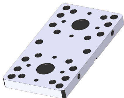
PO-75 BASE AL
